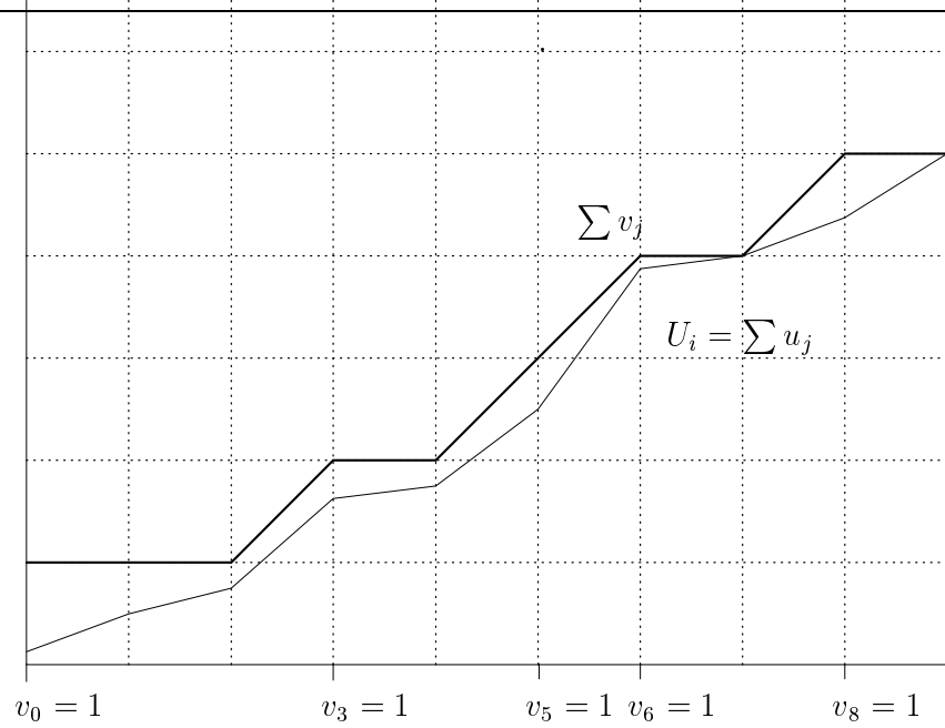
FIG. 6.2 – Exemple de sélection pour laquelle un message sera émis aux instants 0,3,5,6 et 8.
