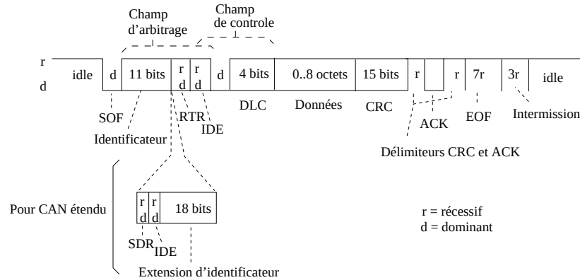
FIG. 1.5 – Format des trames CAN 2.0A et CAN 2.0B au niveau du MAC.
