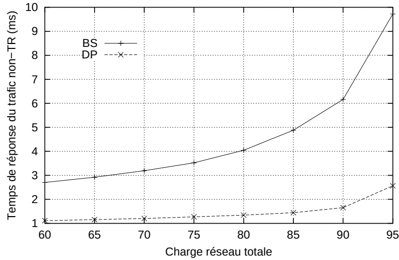
FIG. 5.2 – Temps de réponse moyen du trafic non-TR sous DP et BS.
