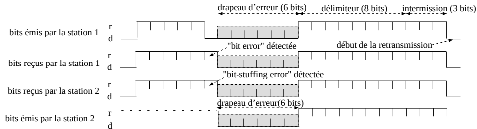
FIG. 1.6 – Détection d’erreur: le cas le plus favorable.
