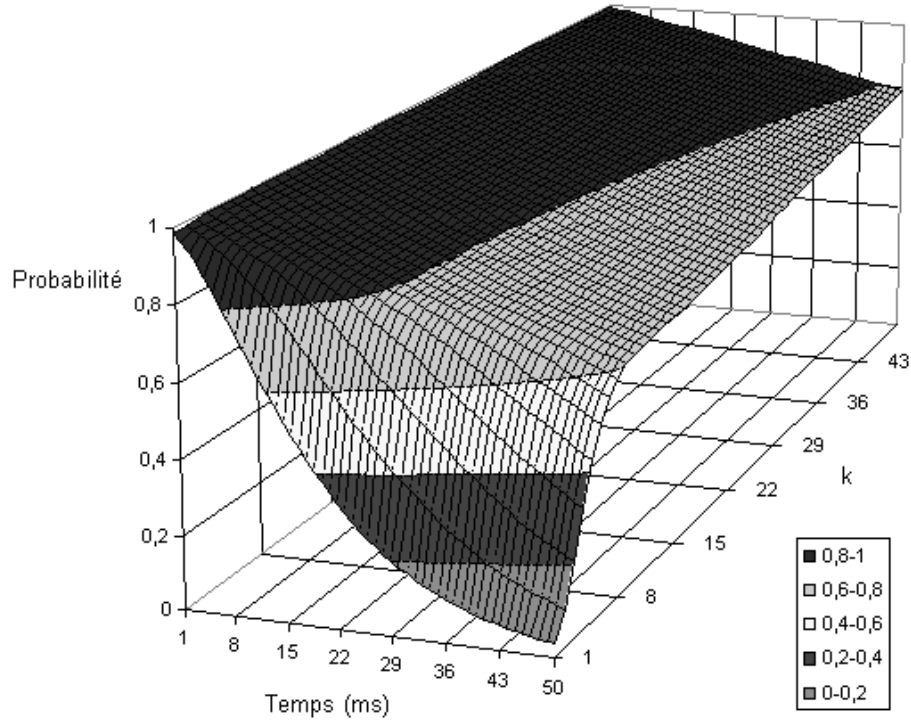
FIG. A.2 – P[X(t) \leq k] avec \alpha = 0.1 , p = 0.04 , \lambda = 100 pour un nombre d'erreurs tolérables k variant de 1 à 50 et pour le temps t variant de 1 à 50 ms.
