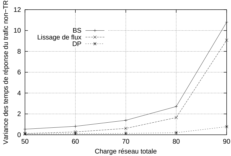
FIG. 6.7 – Variance des temps de réponse du trafic non-TR avec BS, DP et lissage de flux dans le cas désynchronisé.
