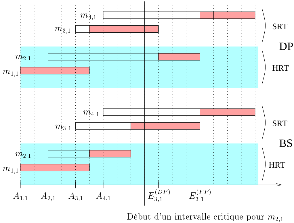
FIG. 5.1 – Une trajectoire sous les politiques DP et BS.
