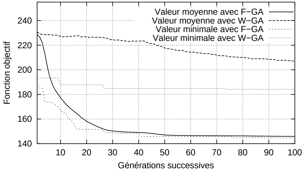
FIG. 4.6 – Évolution de la valeur moyenne et de la valeur minimale de la fonction objectif pendant 100 générations sur un problème à 20 tâches pour F-GA et W-GA.
