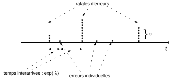
FIG. 2.2 – Le modèle d'erreurs.
