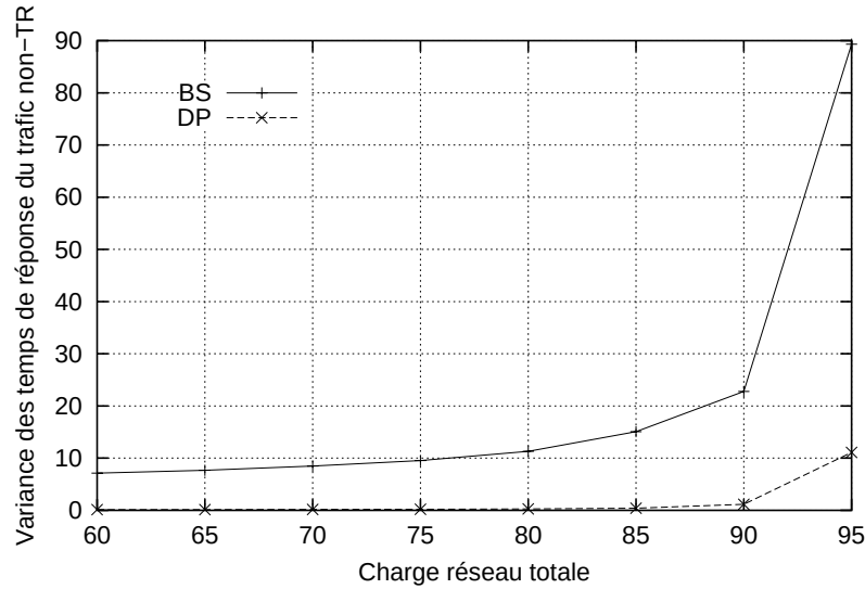
FIG. 5.3 – Variance des temps de réponse pour le trafic non-TR sous DP et BS.
