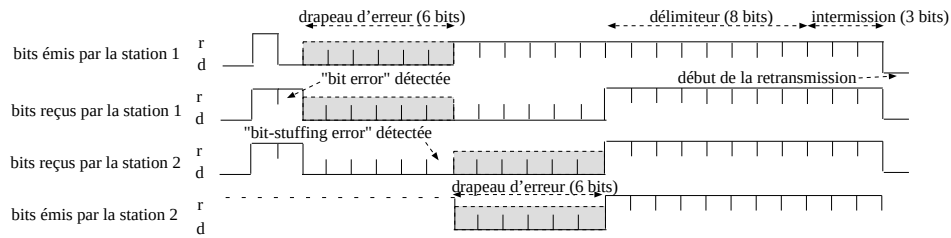
FIG. 1.7 – Détection d'erreur: le pire cas.
